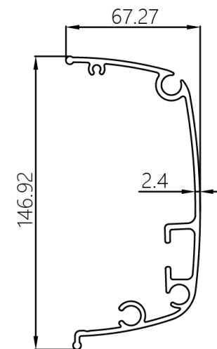
前管
