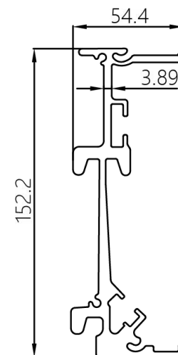
后盒盖
