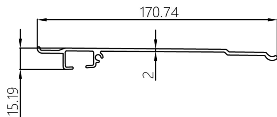
上盒盖
